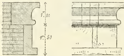
98, 99. — Moulures assyriennes, d'après Botta. Profil et élévation.
